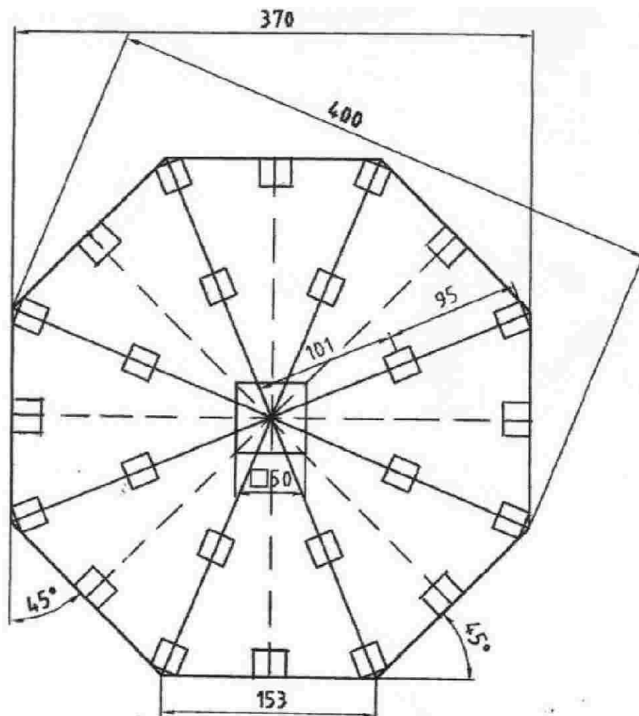
Grundrids Antares Havepavillon
